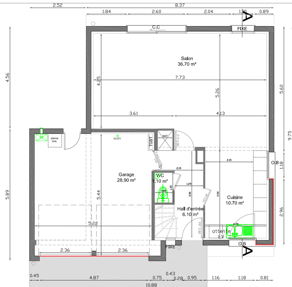
PLAN RDC
