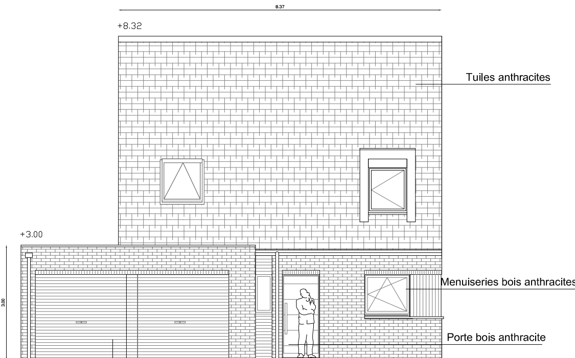
FACADE PRINCIPALE
